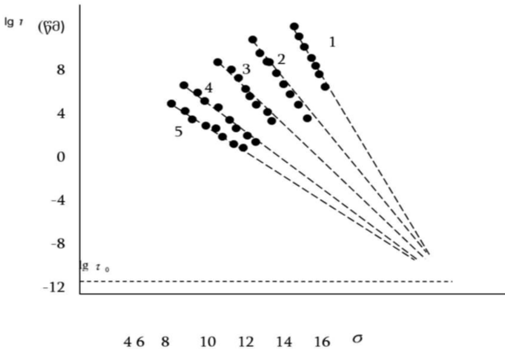
სურ.1. ხანმედეგობის დამოკიდებულება დამაბულობისგან პოლიკაპროამიდისთვის (ორიენტირებული ბოჭკო) სხვადასხვა ტემპერატურებზე
