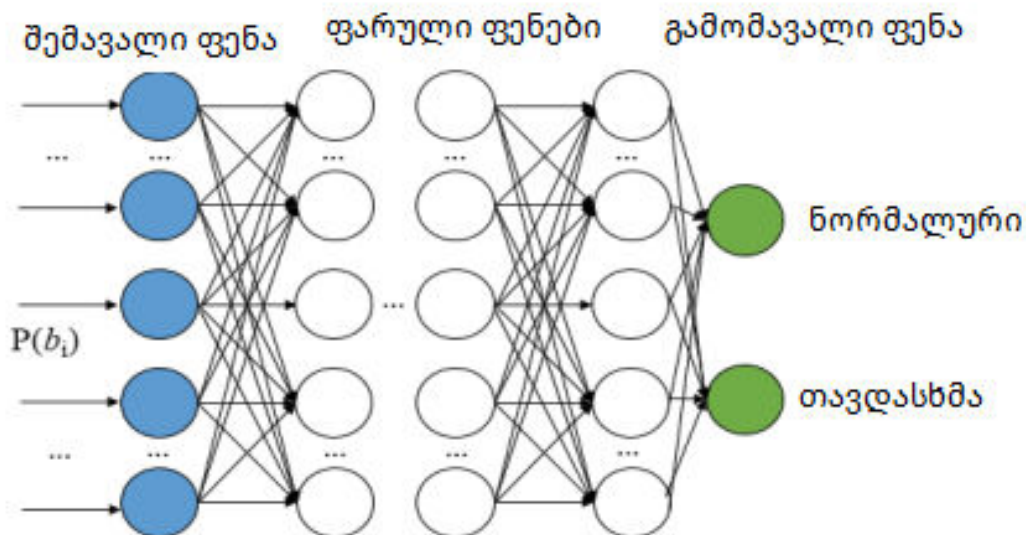
ნახ.4. ნეირონული ქსელის ზოგადი სქემა უსაფრთხოების ამოცანებისთვის
